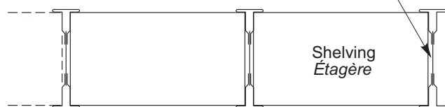
Shelving panel or side braces Entretoise ou panneau d'étagère
